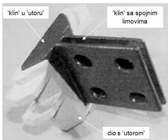
Slika 1 - Dijelovi tipičnog „ATLSS priključka“
