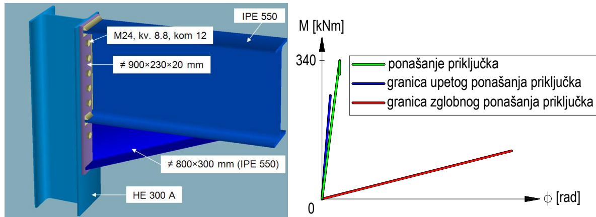
Slika 6 - Suvremeno rješenje priključka prečke i stupa s pripadajućim M - \phi dijagramom (1. varijanta)
