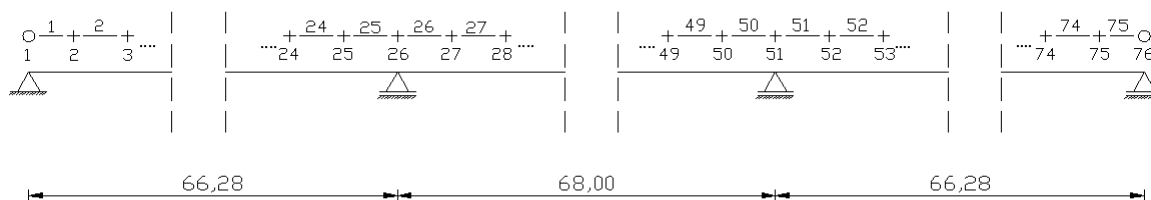
Slika 6 - Raspored čvorova i štapova
