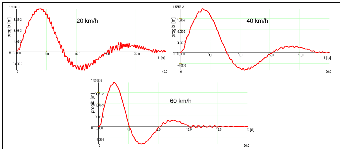
Slika 9 - Grafički prikazi progiba čvora 13 od prelaska kamiona K3
