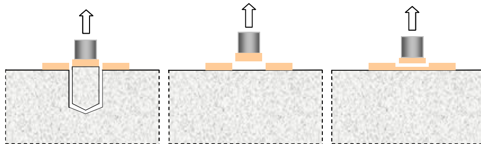
Slika 9 - Različiti modovi sloma betona s površinskom slojem: a) slom u podložnom betonu, b) slom između podložnog betona i površinskog sloja, c) slom u površinskom sloju
