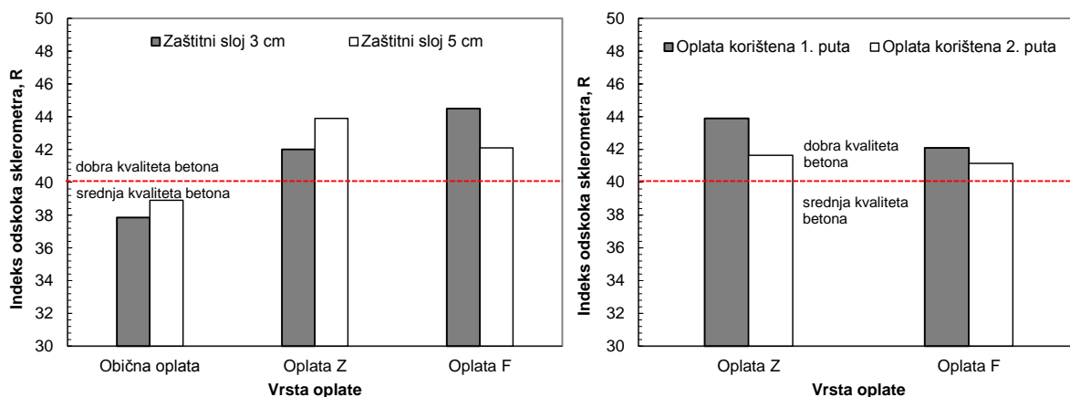
Slika 7 - a) Indeks odskoka sklerometra ispitan na uzorcima sa zaštitnim slojem od 3 i 5 cm; b) Indeks odskoka sklerometra ispitan na uzorcima sa zaštitnim slojem od 5 cm na kojima je oplata drugi puta korištena
