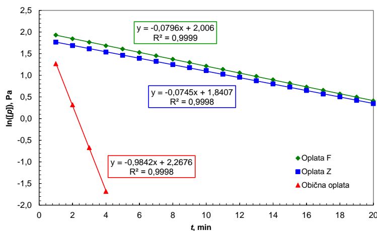
Slika 11 - Promjena pritiska unutar ispitne komore u vremenu tijekom ispitivanja zrakopropusnosti betona pripremljenog u klasičnoj i u CPF oplatama
