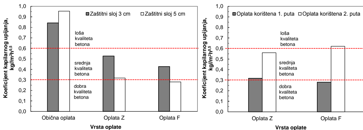
Slika 13 - a) Koeficijent kapilarnog upijanja izračunat za uzorke sa zaštitnim slojem od 3 i 5 cm; b) Koeficijent kapilarnog upijanja izračunat za uzorke sa zaštitnim slojem od 5 cm na kojima je oplata drugi puta korištena
