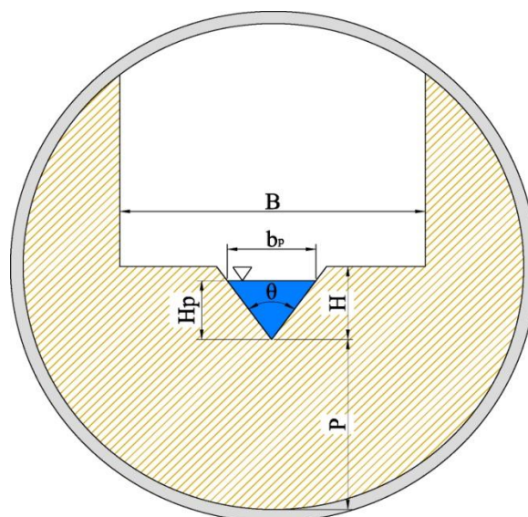
Slika 1 - Trokutni oštrobridni preljev - presjek
