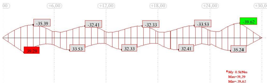
Slika 5 - Anvelopa momenata savijanja oko slabije osi M_{z,Ed} (skupina opterećenja 1, najveći moment oko slabije osi M_{z,Ed} )
